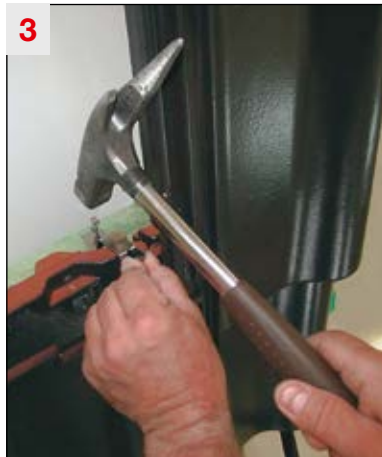
3 ... und von oben in die Traglattung einschlagen.
