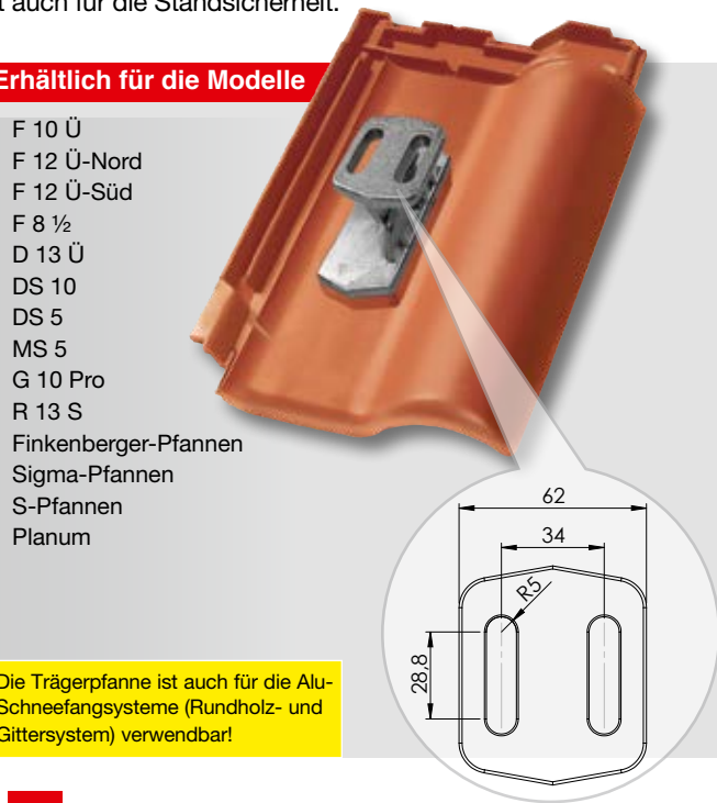
2 Für die Verschraubung in die Traglatte befinden sich zwei Edelstahlschrauben auf der Rückseite der Alu-Solar-Trägerpfanne.
